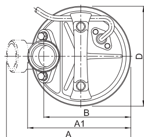
Hrdlo LOT2"-74
