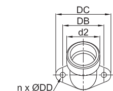
Hrdlo LOT2"-74
